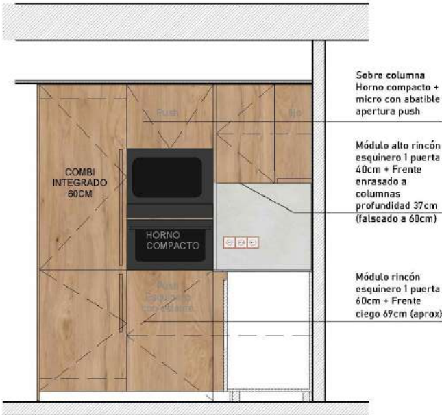
ALZADO LATERAL
