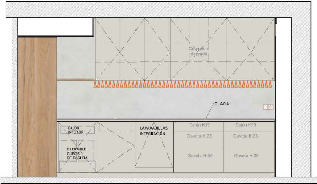
ALZADO FRONTAL
