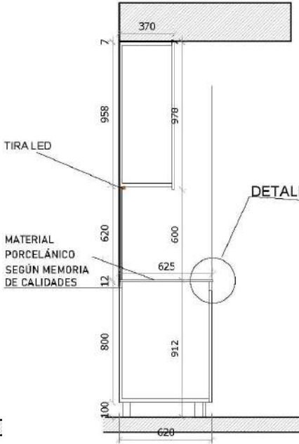
SECCIÓN
